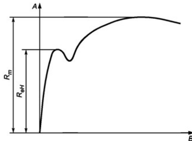
A — предел прочности при растяжении; B — удлинение
