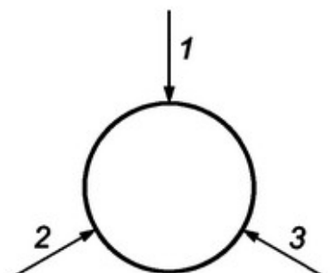
Рисунок 1 — Пример измерения толщины покрытия по окружности стержня
