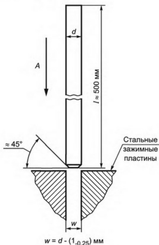
Рисунок 2 — Пример испытания адгезии
