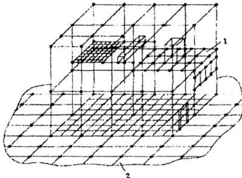
1- сеть соединений; 2 - заземлитель
