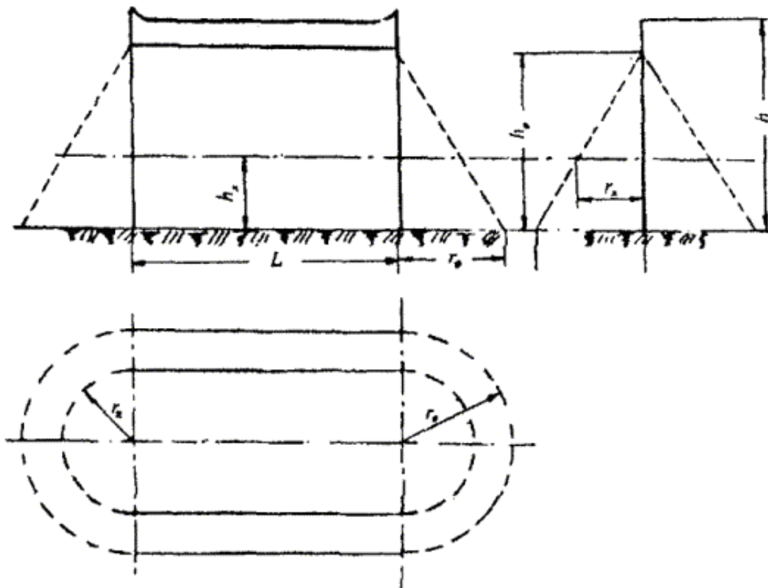
Рисунок 3.2 - Зона защиты одиночного тросового молниеотвода
