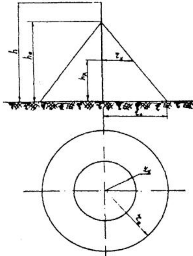
Рисунок 3.1 - Зона защиты одиночного стержневого молниеотвода
