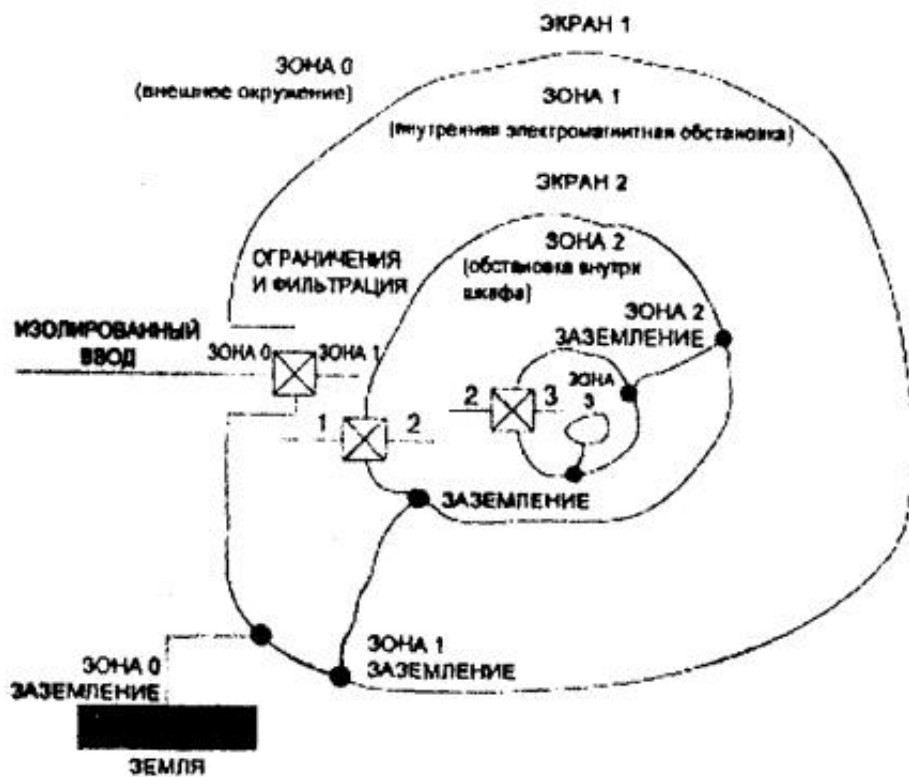
Рисунок 4.1 - Зоны защиты от воздействия молнии
