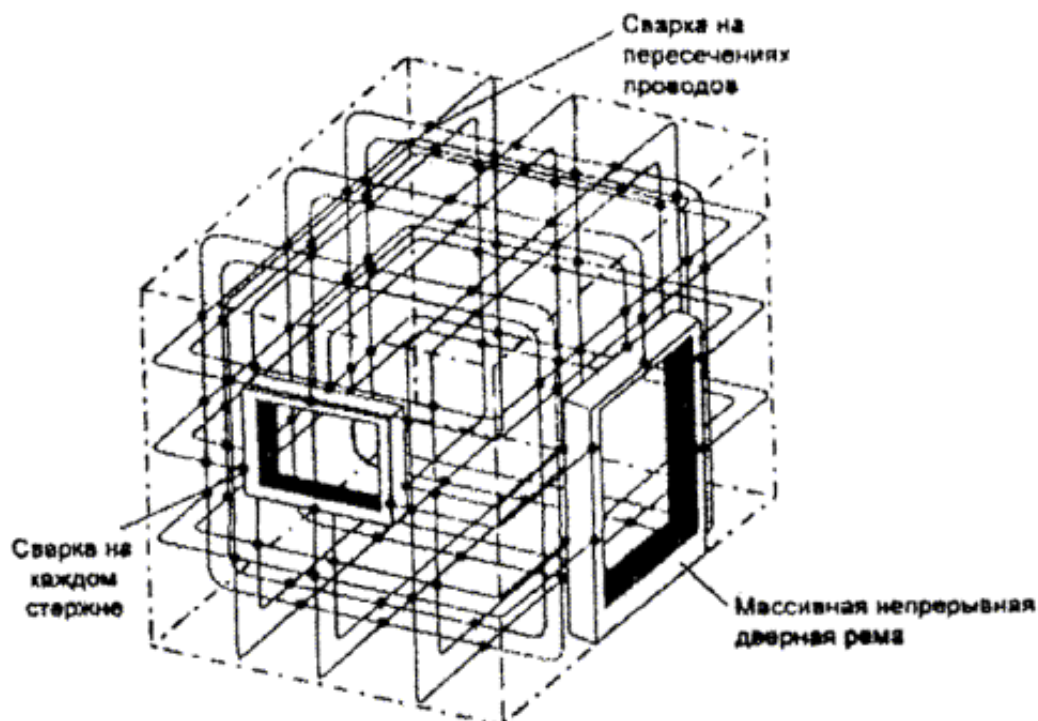
Рисунок 4.3 - Пространственный экран из стальной арматуры
