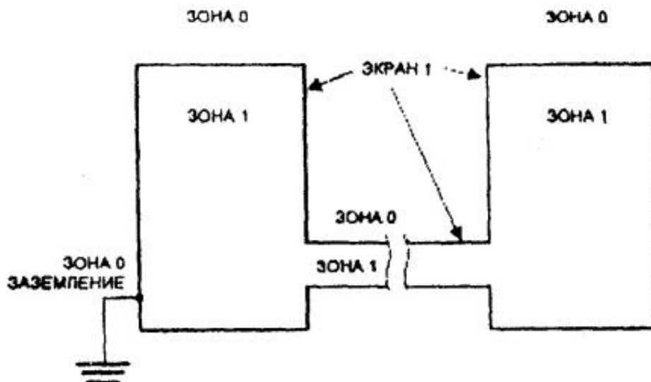
Рисунок 4.2 - Объединение двух зон
