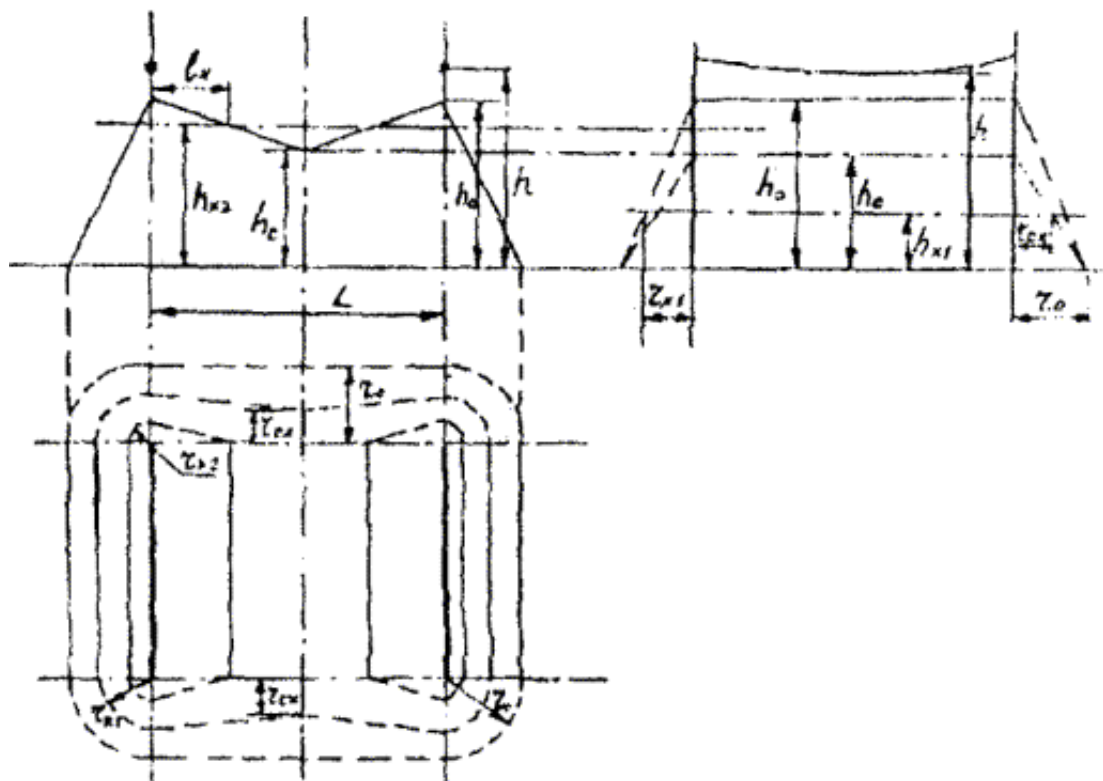
Рисунок 3.4 - Зона защиты двойного тросового молниеотвода
