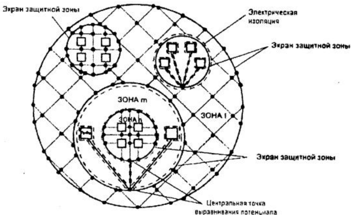
Рисунок 4.6 - Комплексное выполнение системы выравнивания потенциалов
