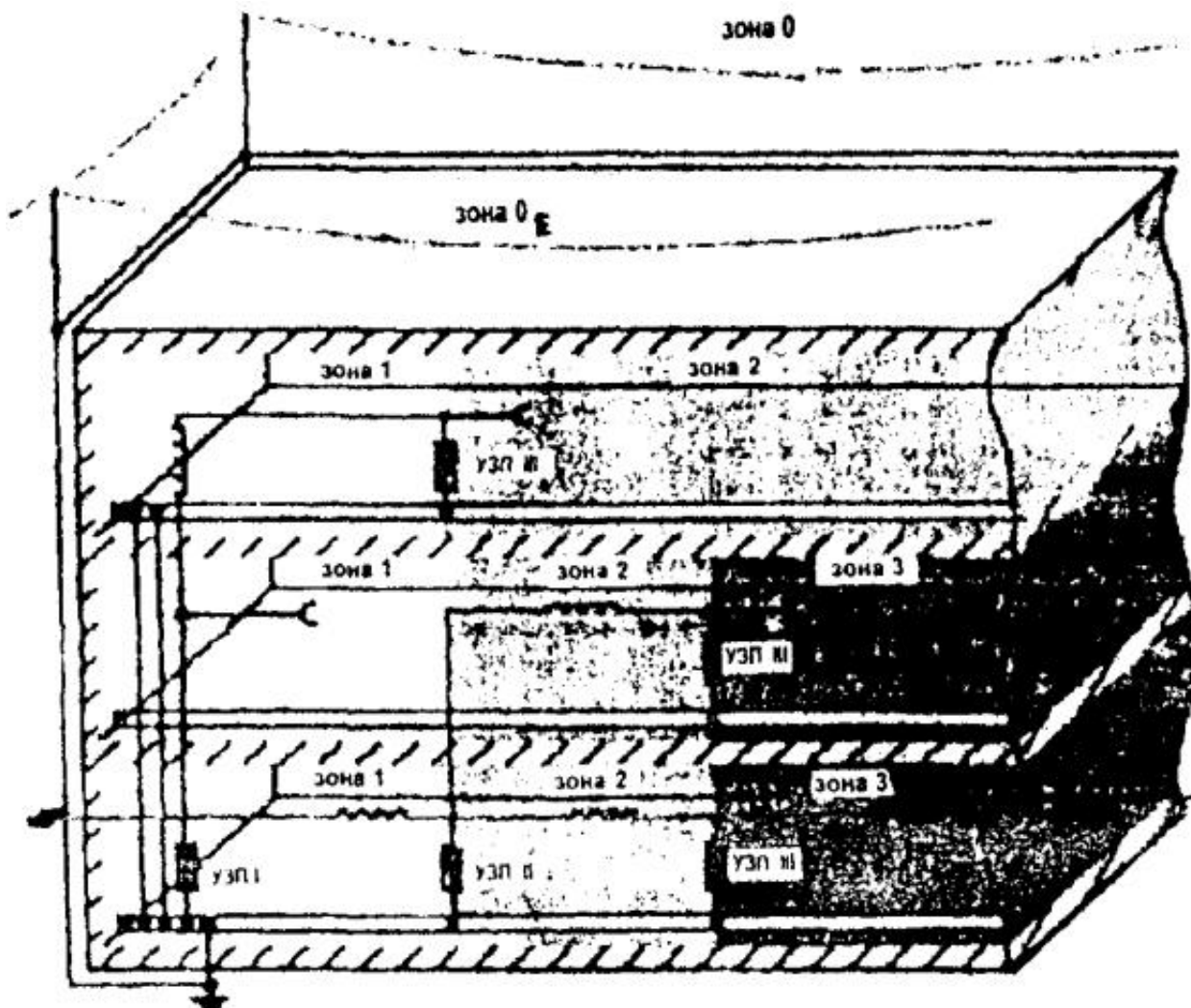
Рисунок 4.9 - Пример установки УЗП в здании
